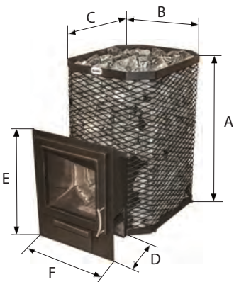
Joonis 13. / Рисунок 13. ST-216, ST-220
