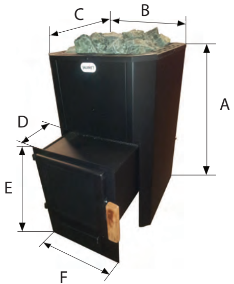
Drawing 4. / Рисунок 4. P-216, P-220
