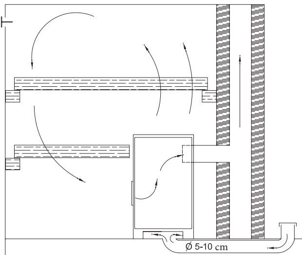
Drawing 1. Natural Ventilation Рисунок 1. Естественная вентиляция
